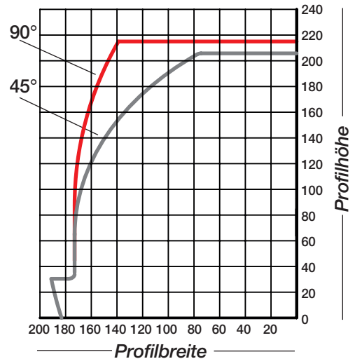
Schnittdiagramm in mm:
