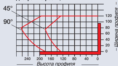
Диаграмма резки, мм:
