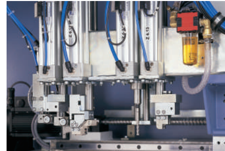
Oberer und unterer Bearbeitungsschlitten mit je 6 Werkzeugplätzen.
