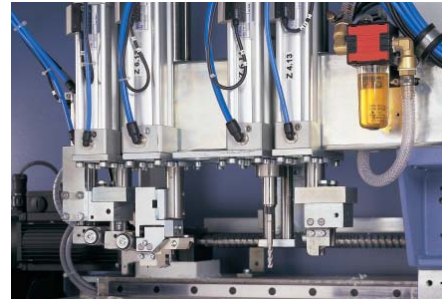
Horné a dolné obrábacie osi z každej strany po 6 miest pre nástroje.
