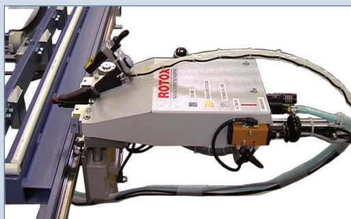
Vorschubschrauber
