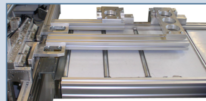
Mjerni graničnik 396-DL sa dva graničnika za 4-struko rezanje
