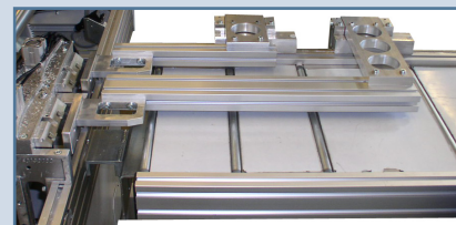
Doraz 396-DL se dvěma dorazy pro 4-nás.řez
